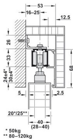
Wandmontage met wandbeugel & bevestigingsclip voor houten afwerking naar keuze
