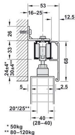
Wandmontage met profiel onzichtbare wandmontage deuren 28-40mm dik
