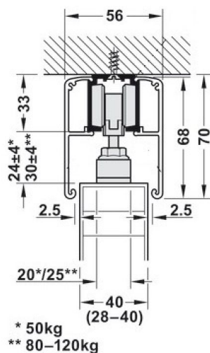
Plafondmontage met 2 maal afdeklijst
