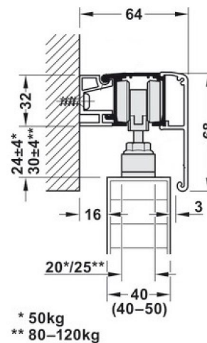
Wandmontage met profiel onzichtbare wandmontage deuren 40-50mm & afdeklijst
