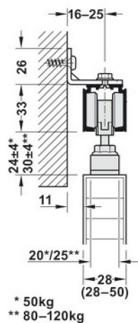
Wandmontage met wandbeugel & bevestigingsclip voor houten afwerking naar keuze
